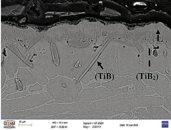
Şekil 4. Borlanmış Grade 5 titanyum alaşımının yüzeyinde oluşan çift fazlı tabakanın taramalı elektron mikroskobundan (SEM) alınan görüntüsü.
