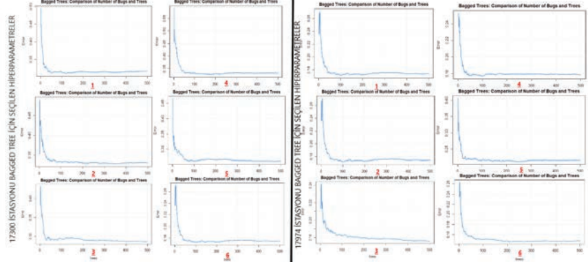
Şekil 7. Bagged Tree optimum hiperparametre değerleri
