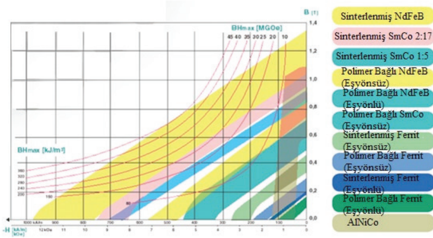
Şekil 4. Çeşitli sabit mıknatısların demanyetizasyon eğrileri (Sura Magnets, 2021)
