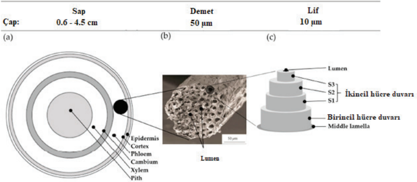
Şekil 3. Kenevir lifinin yapısı: (a) enine kenevir sapı bölümü, (b) kenevir lifi demetinin enine kesit morfolojisi ve (c) kenevir temel lifinin şematik tasviri
