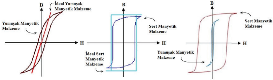
Şekil 1. Sert ve yumuşak manyetik malzeme histerezis eğrisi (Furlani, 2001)
