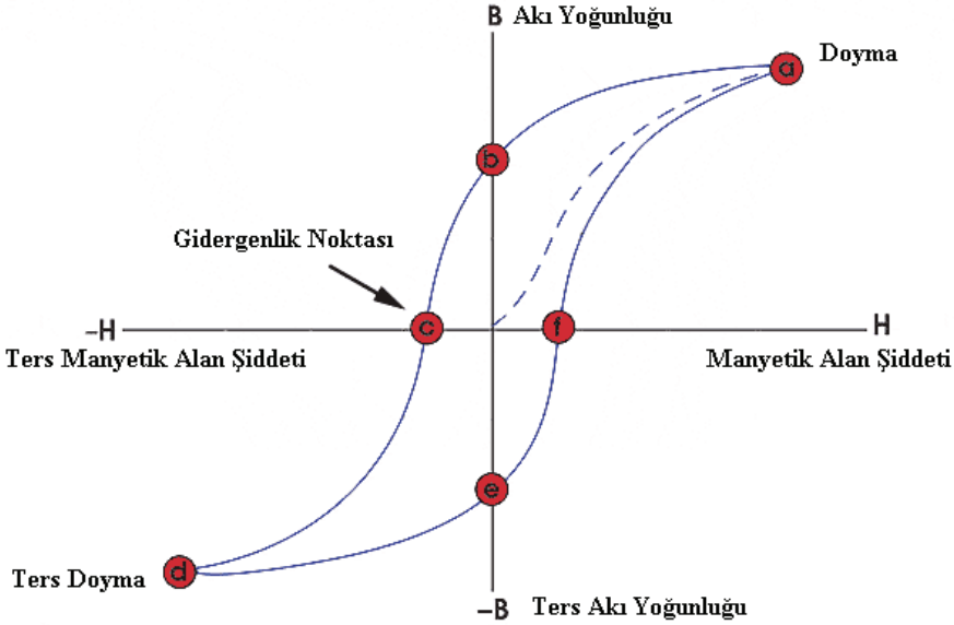
Şekil 2. Sabit Mıknatıs Histerezis Eğrisi (Furlani, 2001)
