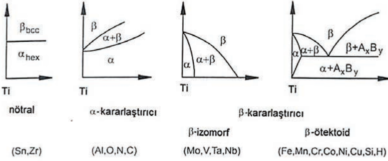
Şekil 2. Alaşım elementi ilavesinin titanyum faz diyagramına etkisinin şematik gösterimi [4].
