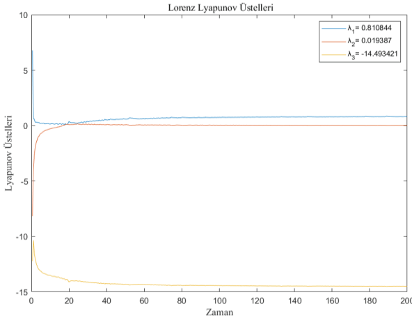
Şekil 2. Lorenz dinamik sisteme ait Lyapunov üstelleri.
